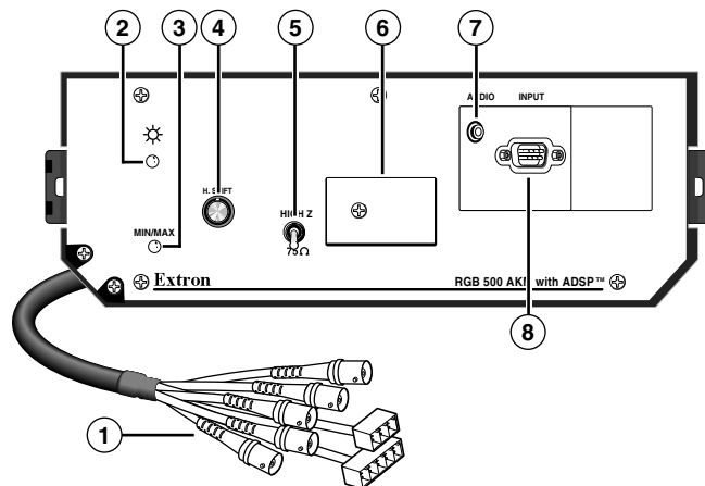
Abbildung 2 — Bedienungsfeld des RGB 500 AKM
