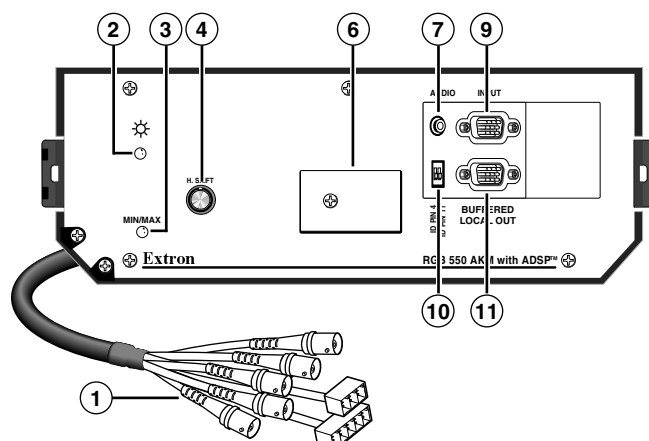
Abbildung 3 — Bedienungsfeld des RGB 550 AKM
