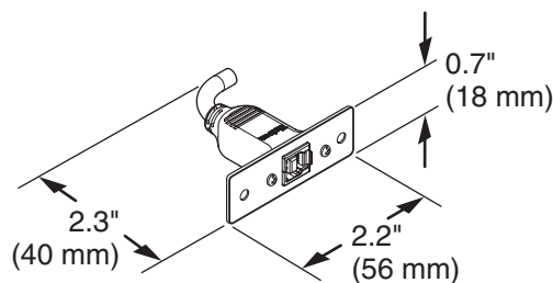
USB B
