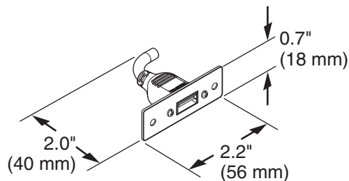
USB A
