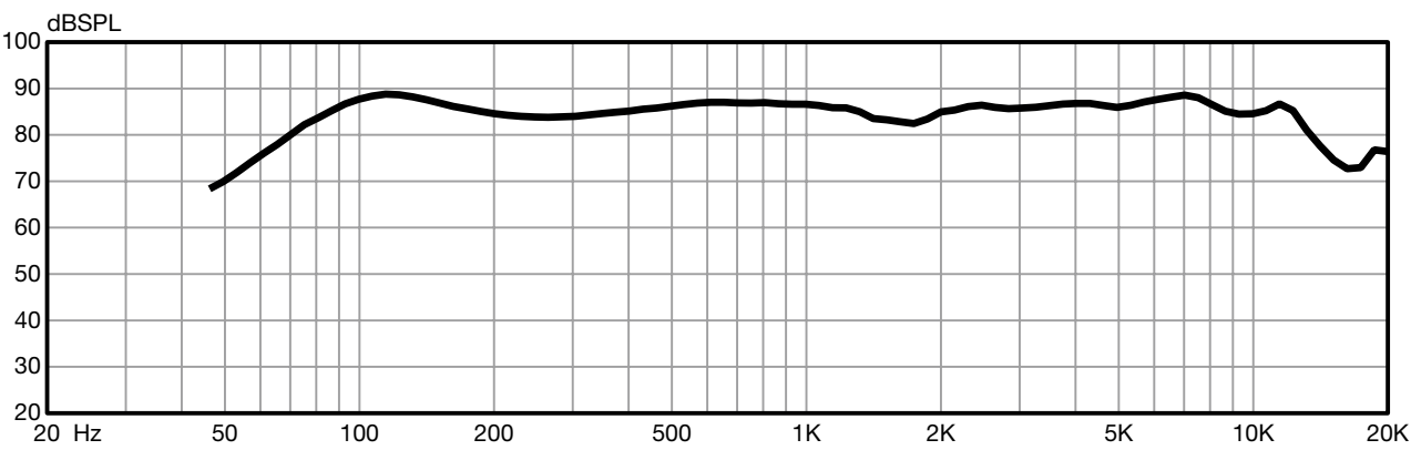
SPL VS. 频率 – 1 W, 1 M 响应, 全空间 (4π)
