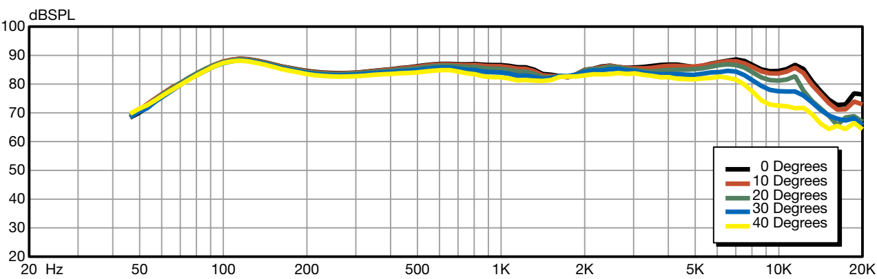
SPL VS. 频率 – 离轴响应, 全空间 (4π)
