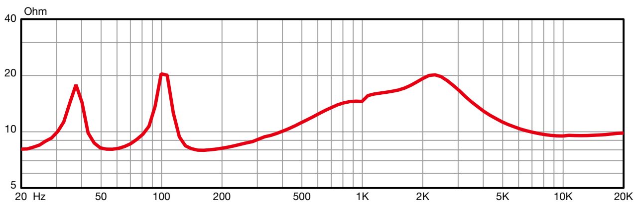
阻抗与频率
