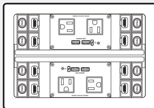
带四单元安装套件的 Cable Cubby 1400; 需要两个 也提供带三单元安装套件的型号; 需要两个
