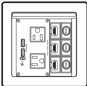
带三单元安装套件的 Cable Cubby 500
