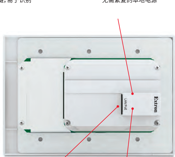
NBP 200 - 后面板
