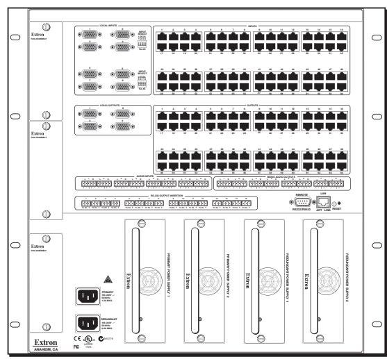
后面板
