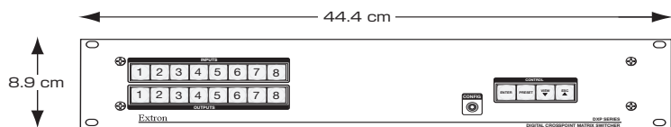
DXP DVI Pro - 前视图
