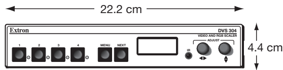
DVS 304 DVI D - 前视图
