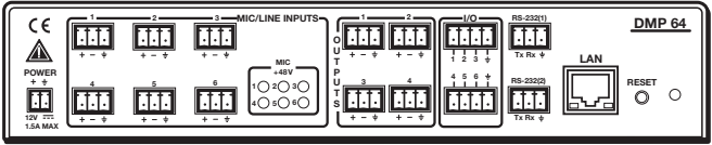
DMP 64 - 后视图
